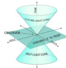
Σχήμα 3.1: Κώνος φωτός
