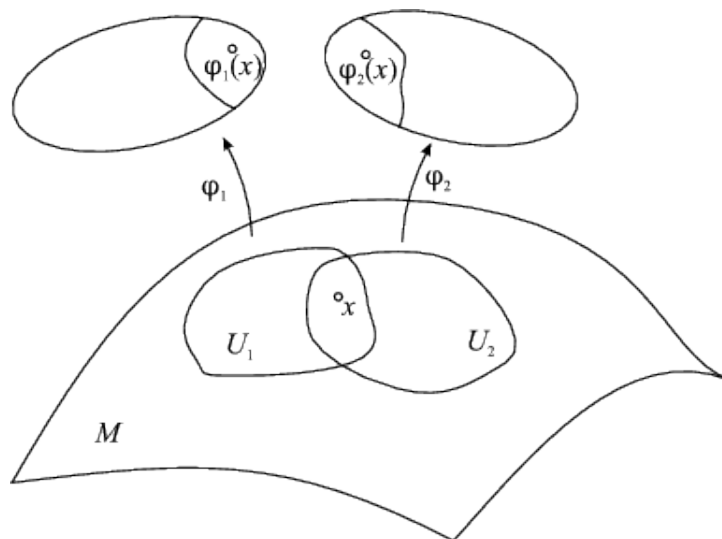
Σχήμα 1.1: Διαφορίσιμη πολλαπλότητα
