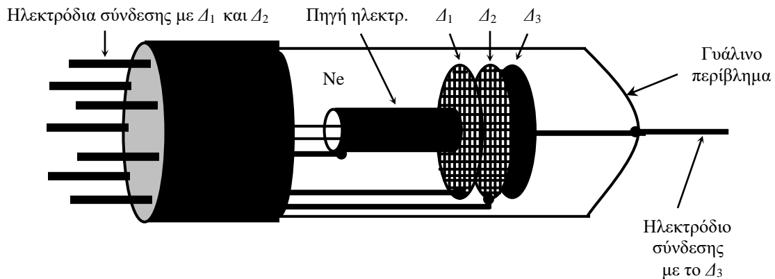
Σχήμα 33.3. Λυχνία Νέου
